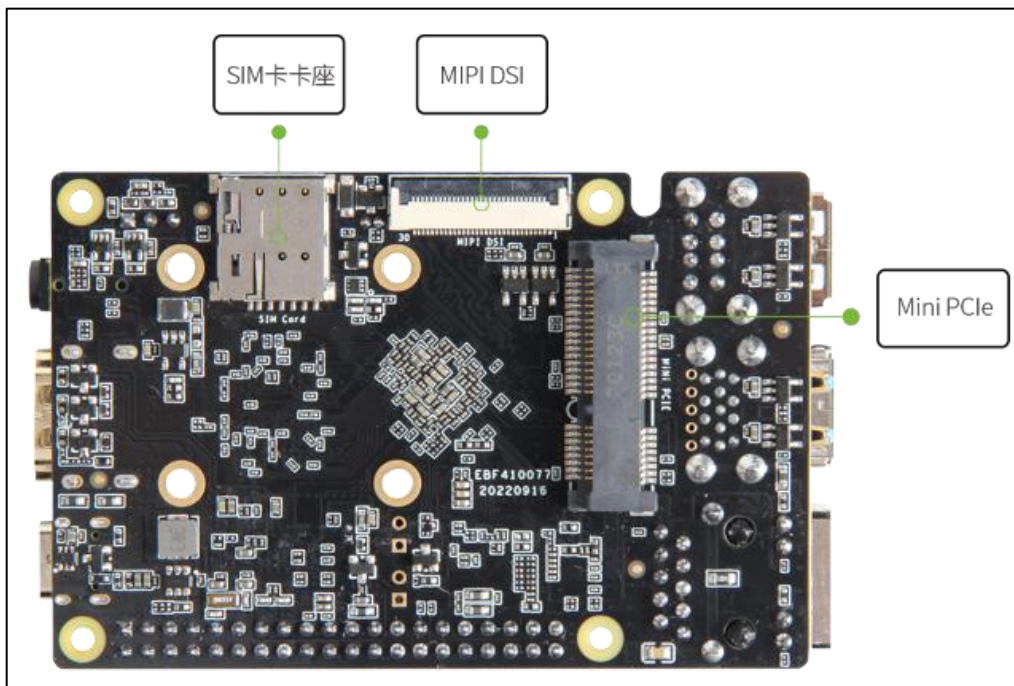
图 3.2.1-3 鲁班猫 1 背面视图
