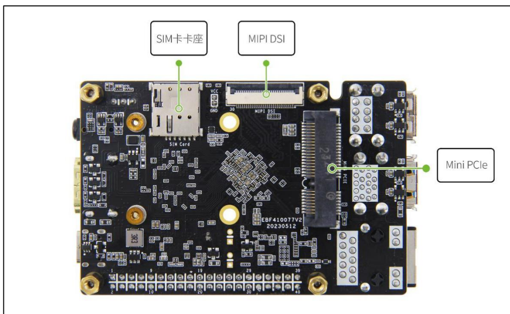
图 3.2.1-6 鲁班猫 1-V2 背面视图
