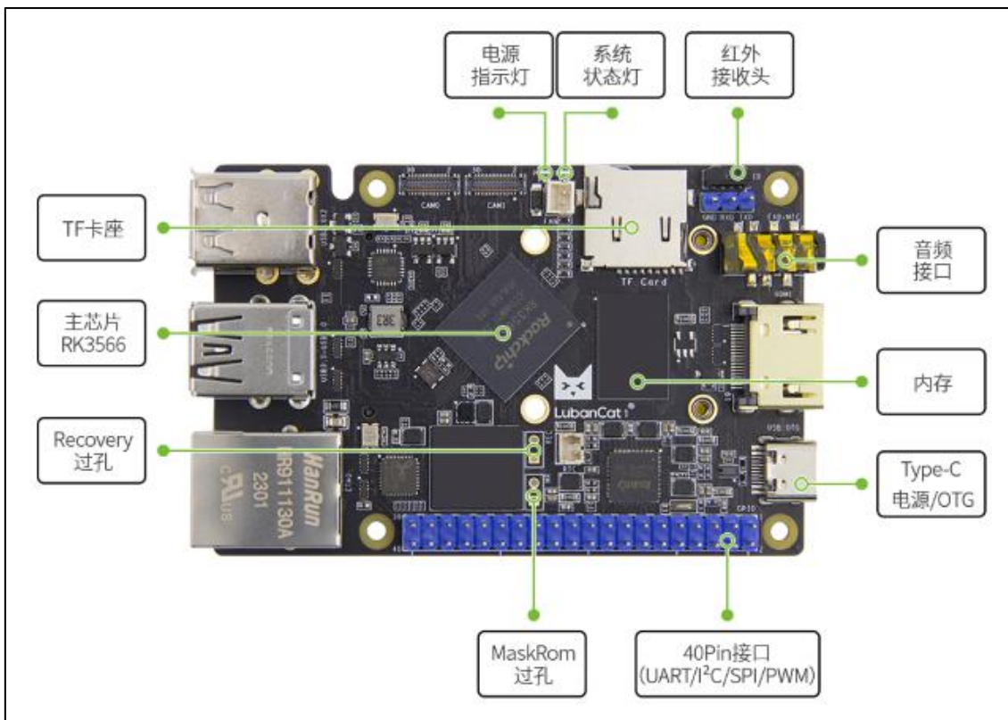
图 3.2.1-5 鲁班猫 1-V2 正面视图 2
