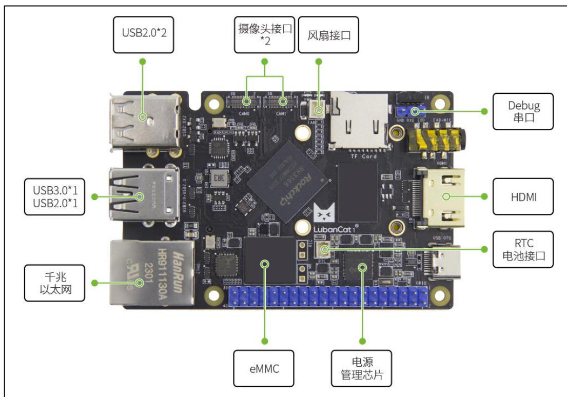
图 3.2.1-4 鲁班猫 1-V2 正面视图 1
