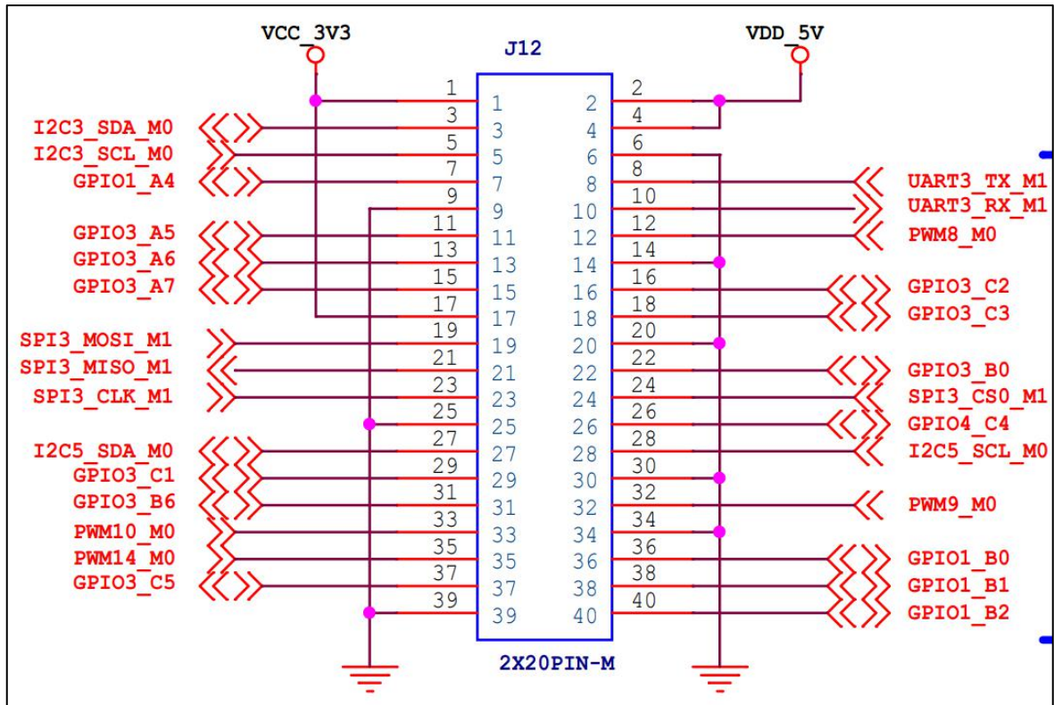
图 4.4-1 鲁班猫 1 系列引脚原理图
