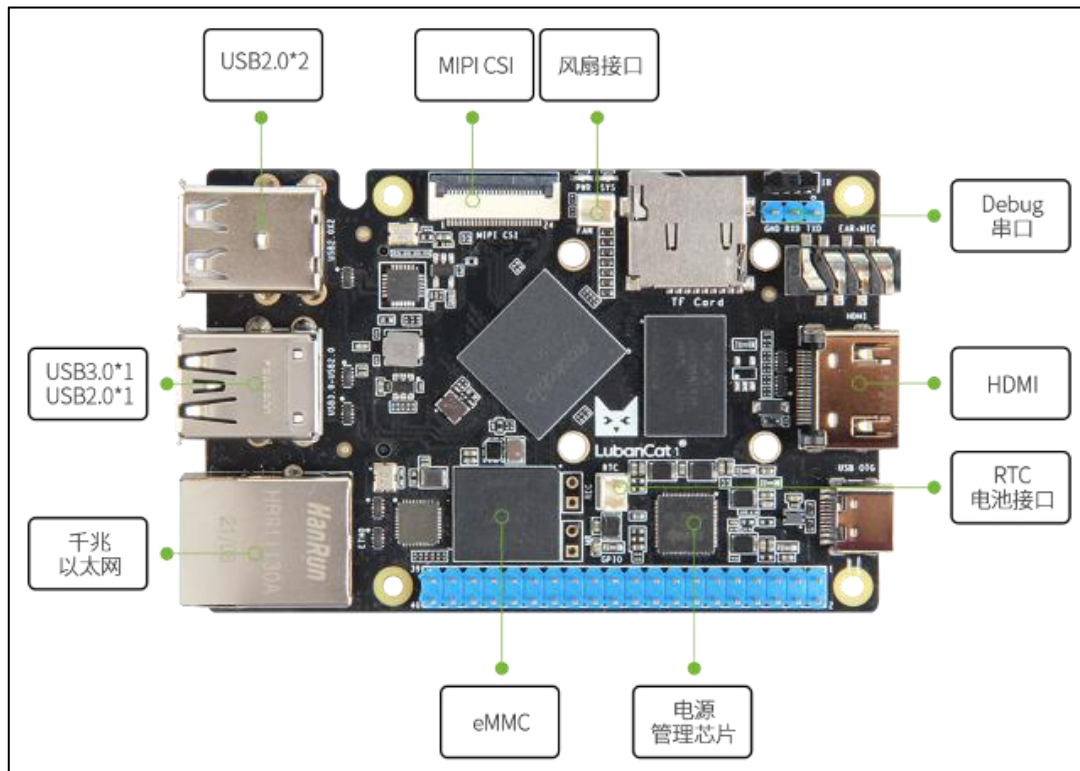
图 3.2.1-1 鲁班猫 1 正面视图 1
