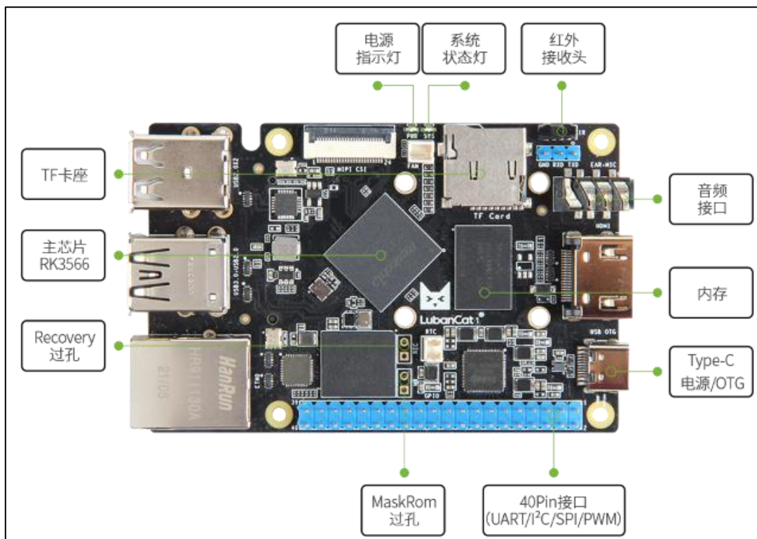
图 3.2.1-2 鲁班猫 1 正面视图 2
